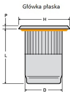
NITONAKRĘTKA M10 z uszczelnieniem PVC 080576 ALS3T-1015-7,9BS
