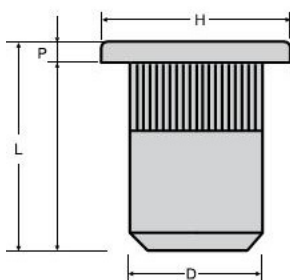
Nitonakrętka M8 ze stali nierdzewnej A2
