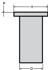
Nitonakretka neoprenowa M4 x 12,6 z gwintem mosiężnym
