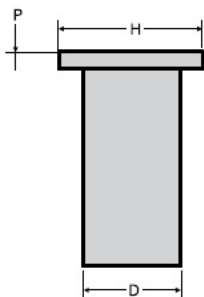
Nitonakrętka neoprenowa M5 x 17 z gwintem mosiężnym
