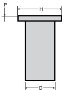
Nitonakrętka neoprenowa M5 x 21,5 z gwintem mosiężnym
