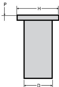
Nitonakrętka neoprenowa M6 x 16 z gwintem mosiężnym
