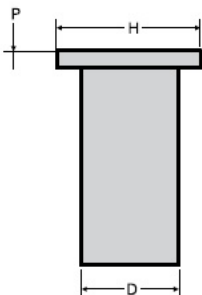
Nitonakrętka neoprenowa M6 x 26,7 z gwintem mosiężnym
