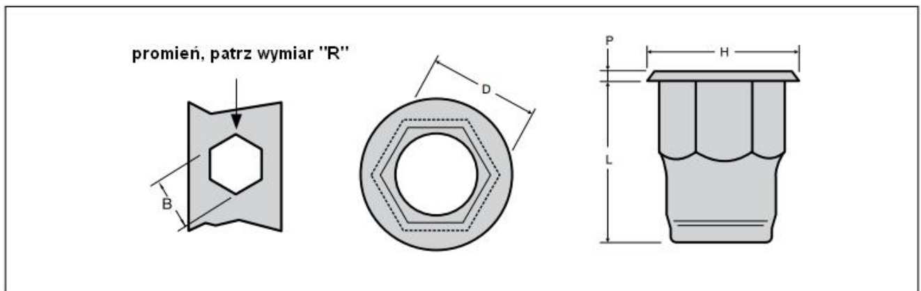
Nitonakrętka sześciokątna M4 seria A-H
