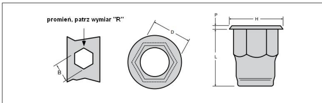
Nitonakrętka
